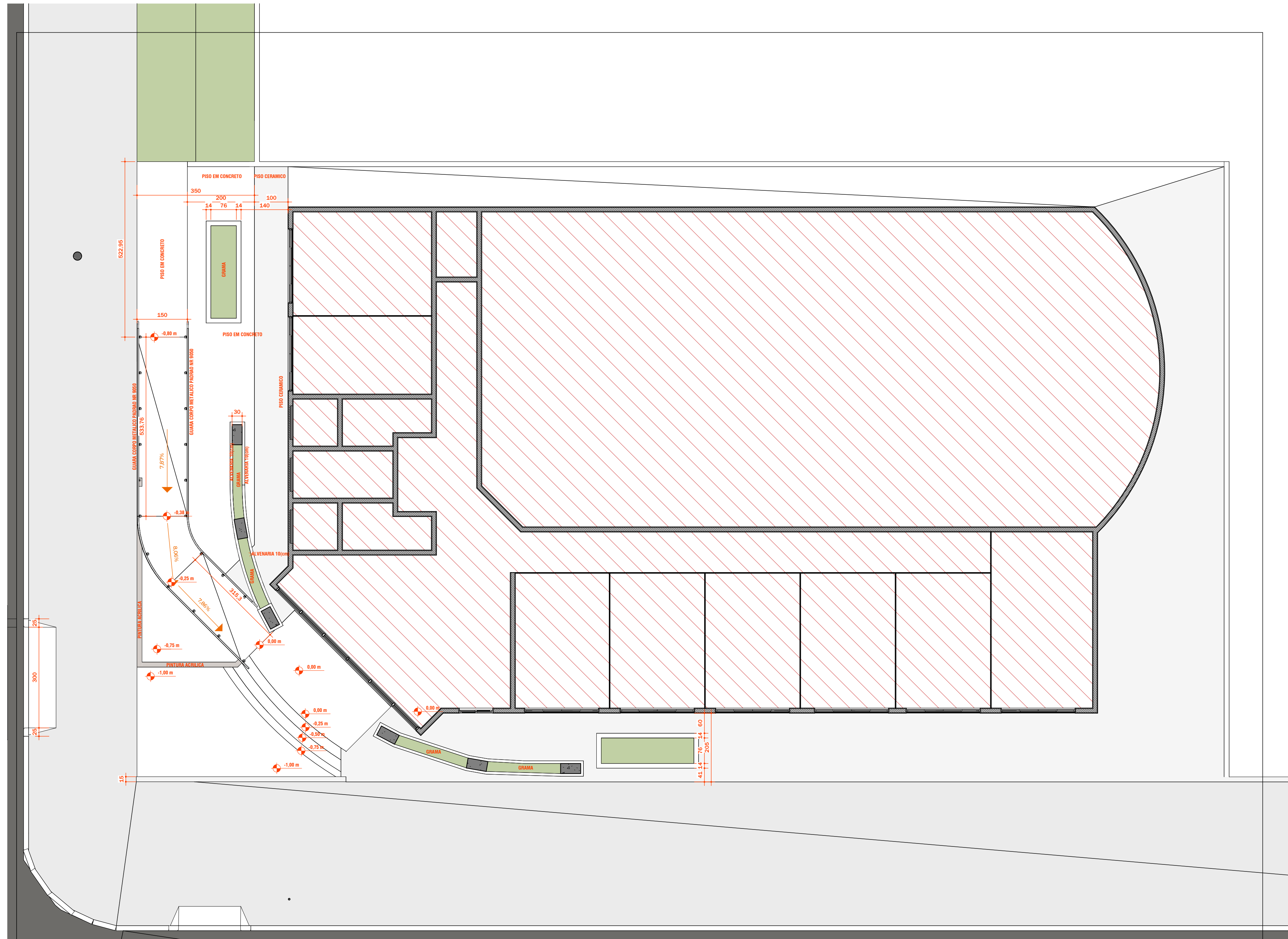
1- 610.TÉRREO Escala 1:75
